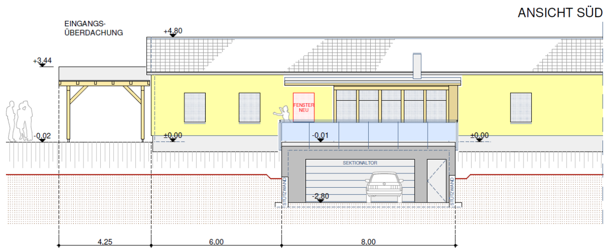
Ansichten Haupthaus: Süd und Ost
