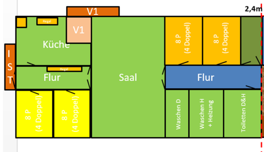
Grundriss Hauptgebäude; Erdgeschoss – neue Raumaufteilung im vorderen/nördlichen Teil des Hauptgebäudes
